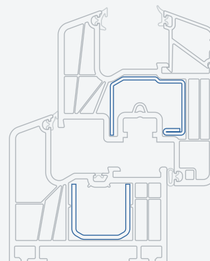
Prestige s rovným krídlom I 76.6 C2 s dorazovým tesnením (AD)
