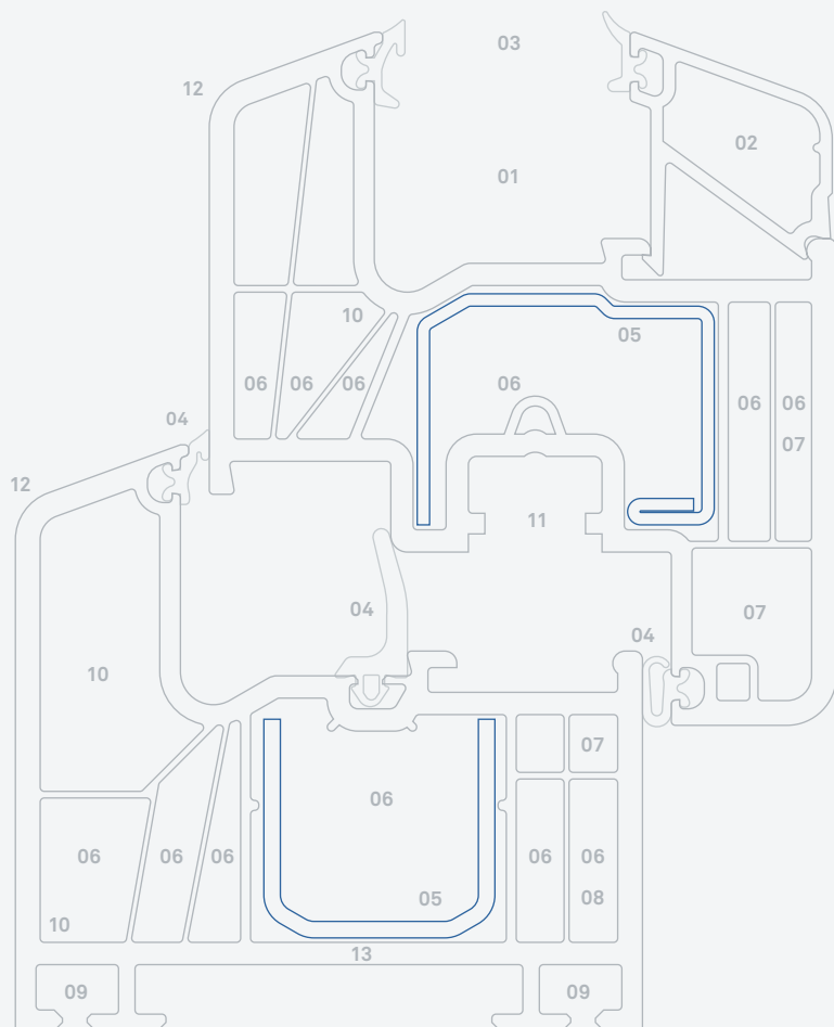
Prestige s rovným krídlom I 76.6 C2 so stredovým tesnením (MD)
